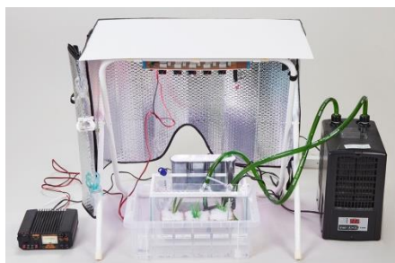
恩賜記念賞 アマモの発芽・育成装置及び方法
